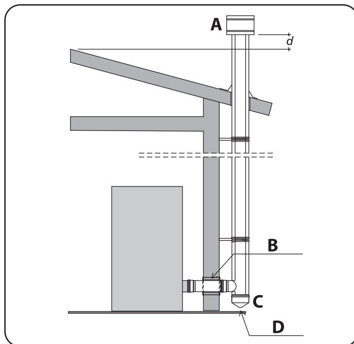
A. SOMBRETE ANTIVIENTO B. AISLAMIENTO C. INSPECCIÓN D. DESCARGA CONDENSACIONES
