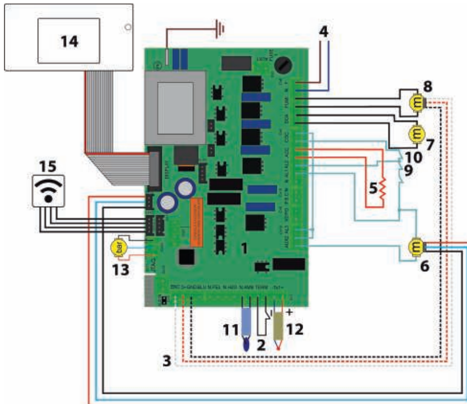
LEYENDA ESQUEMA PRÁCTICO DEL CONJUNTO
